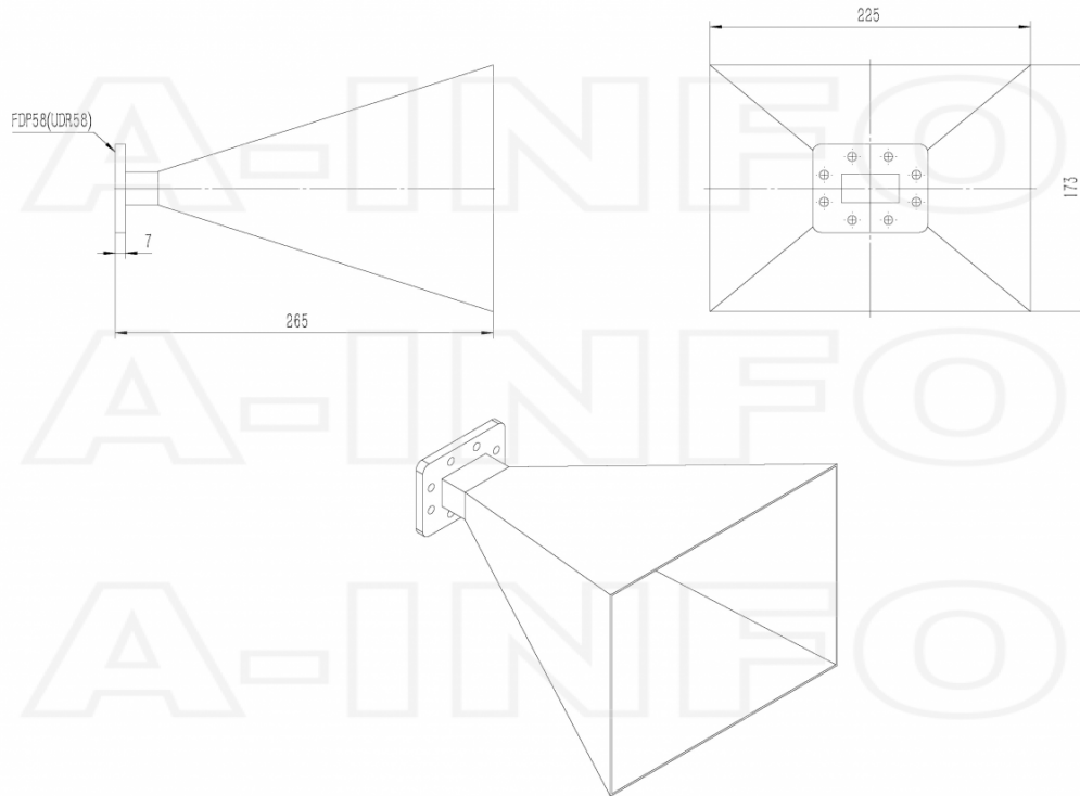
FDP58 Output (P/N: LB-159-20-A)
